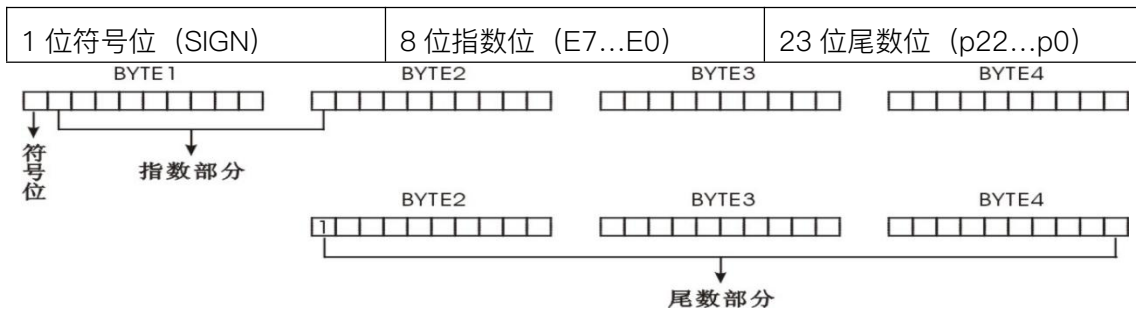
32 浮点型 IEEE-574 数据格式定义
