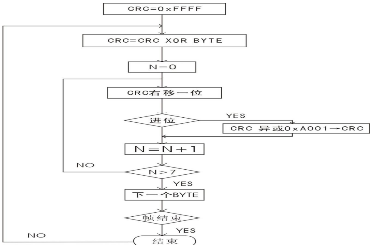
CRC16 校验码计算程序流程图
